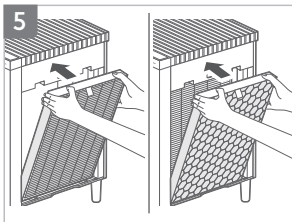
새로운 탈취필터/초미세먼지 집진필터 교체하기
