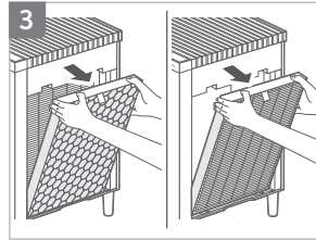
탈취필터/초미세먼지 집진필터 분리하기
